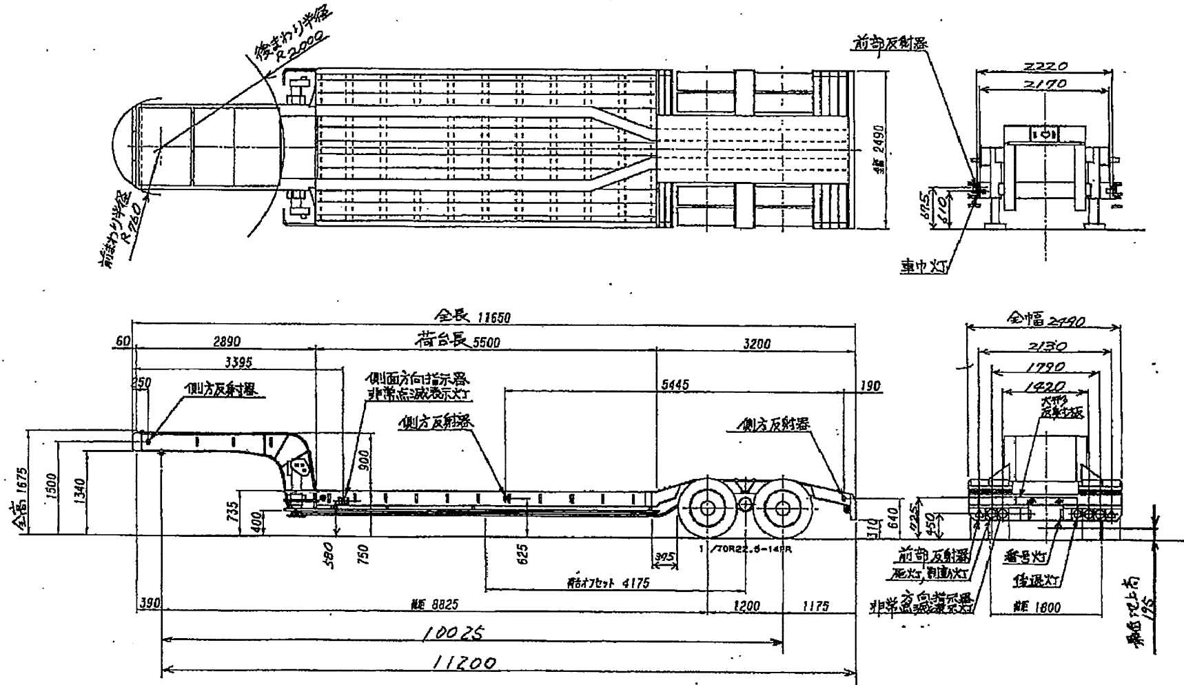
トレーラモビル PMR238AA型 外形四面図
